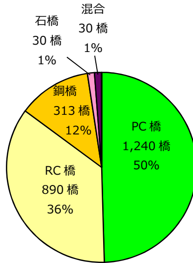
図 - 橋種別の橋梁数
