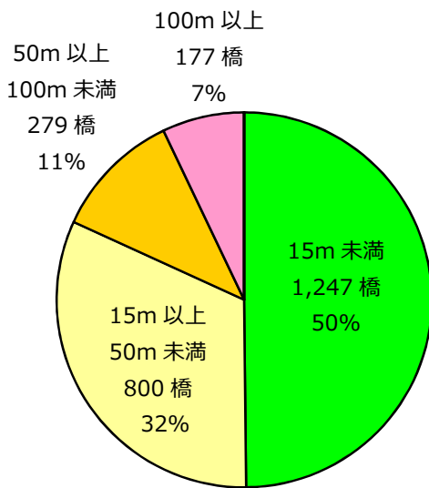
図 - 橋長別の橋梁数
