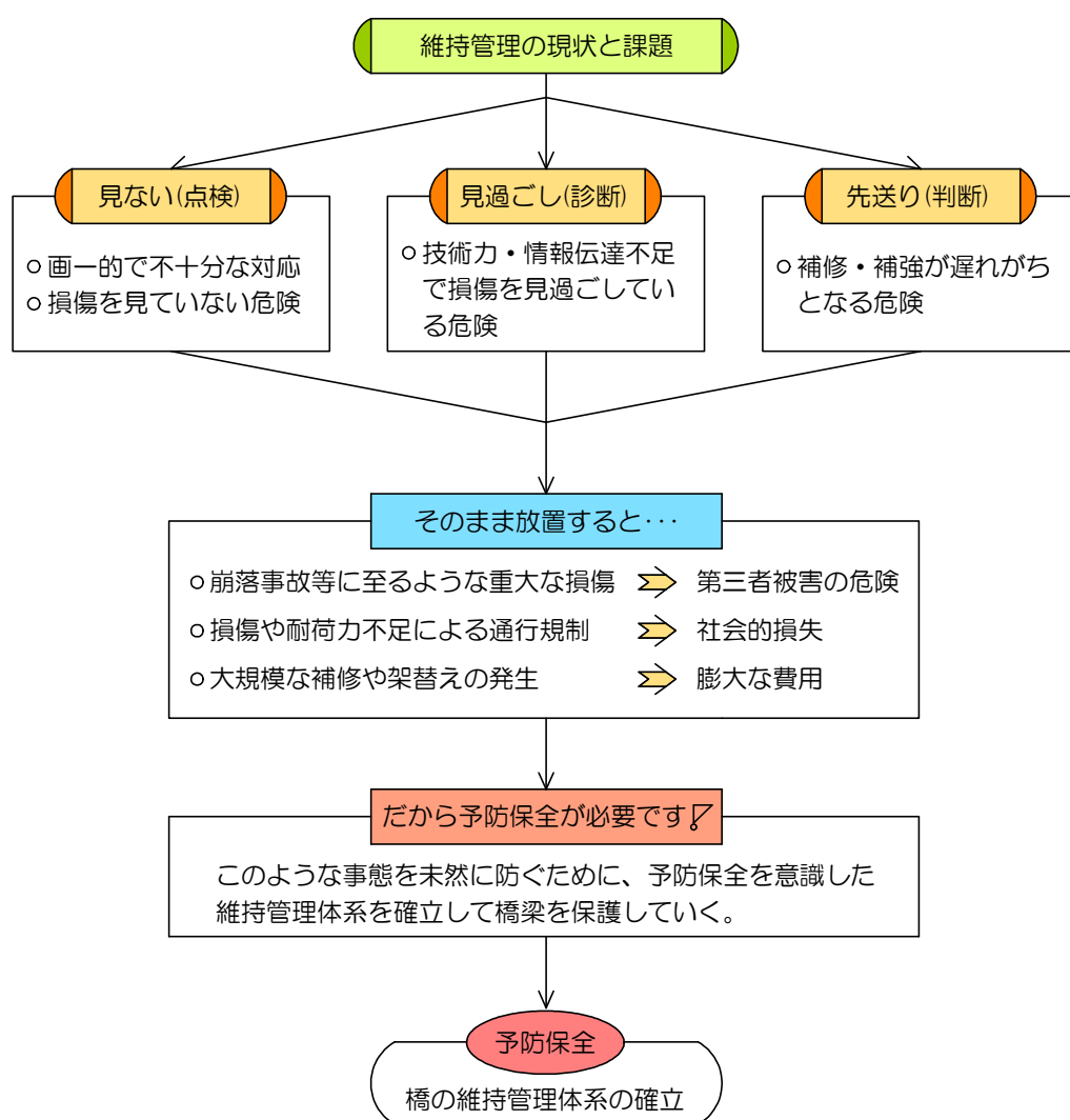
図一 予防保全の流れ
