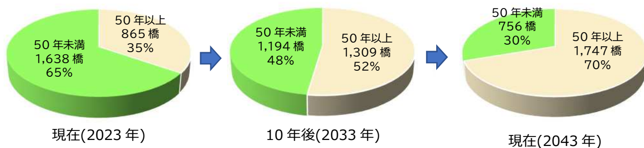
図－建設後50年以上となる橋梁の割合
