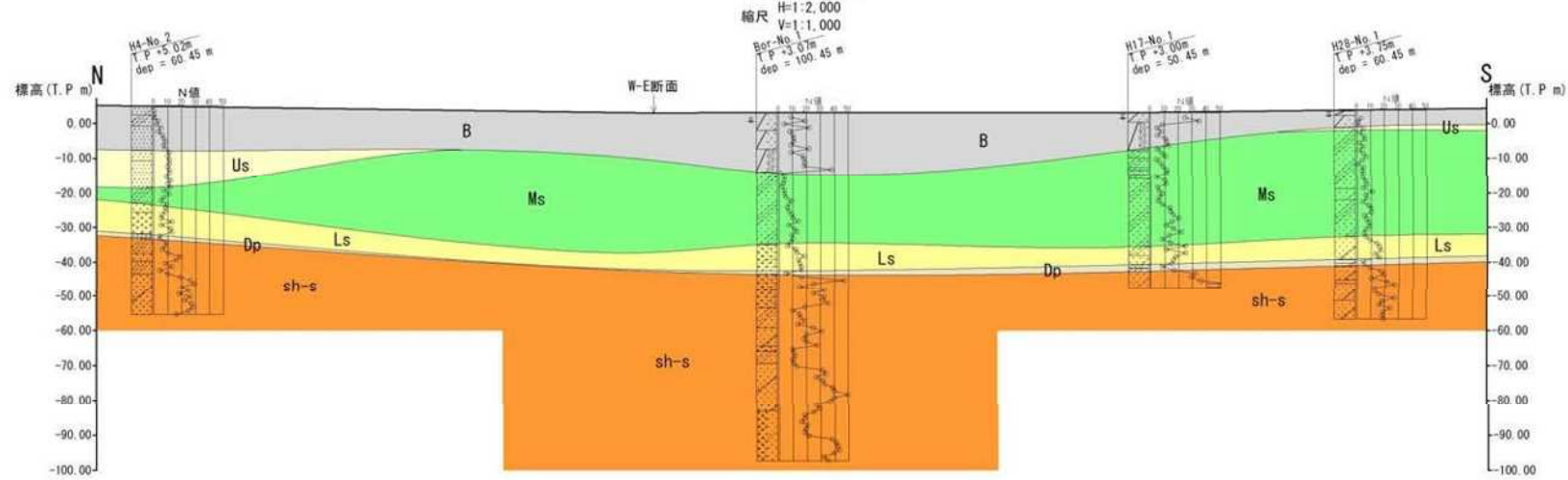
N-S 地質断面図
